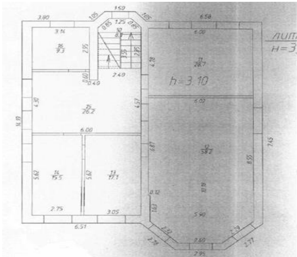
Позтажний план жилого дома, согласно БТИ 1 этаж:
