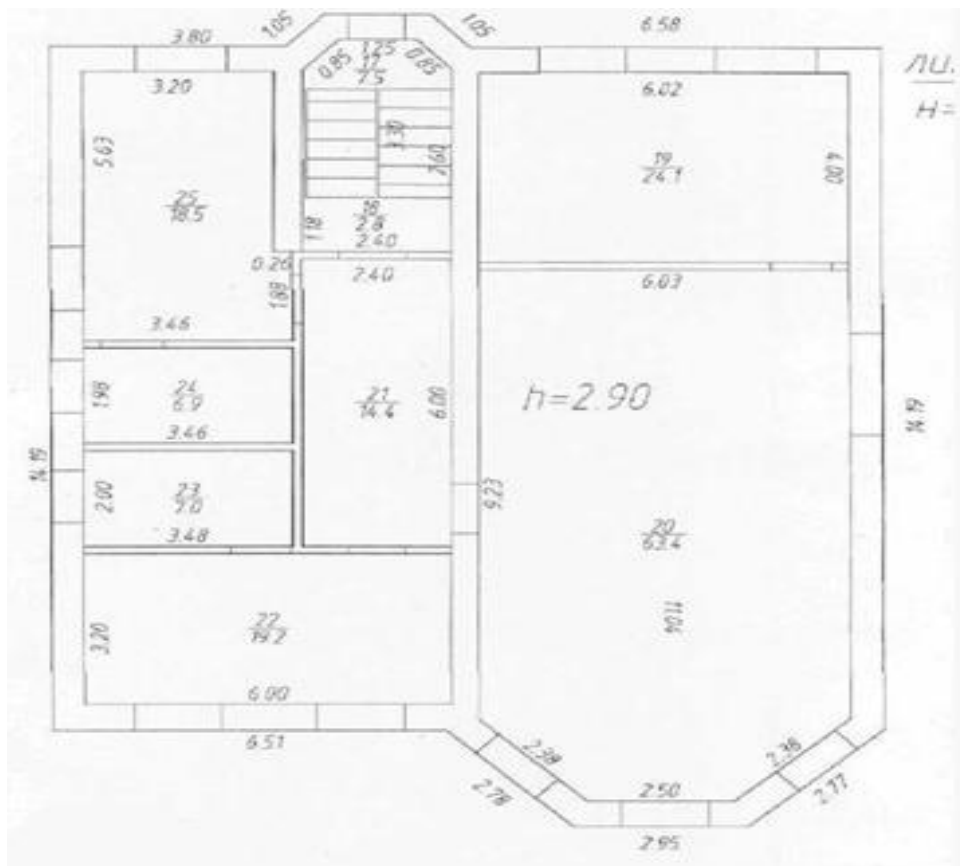
Поэтажный план жилого дома, согласно БТИ 2 этаж:
