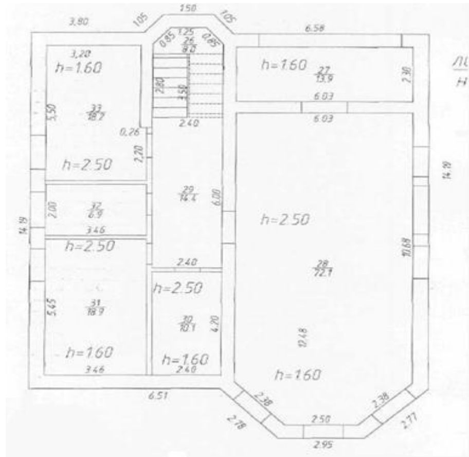
Поэтажный план жилого дома, согласно БТИ мансардный этаж:
