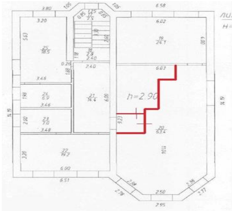
Фактический поэтажный план жилого дома, 2 этаж:
