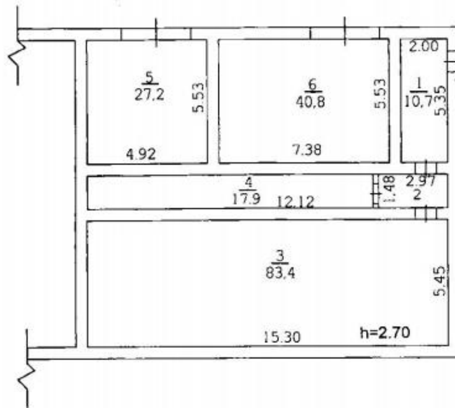
Лит.А План подвала
